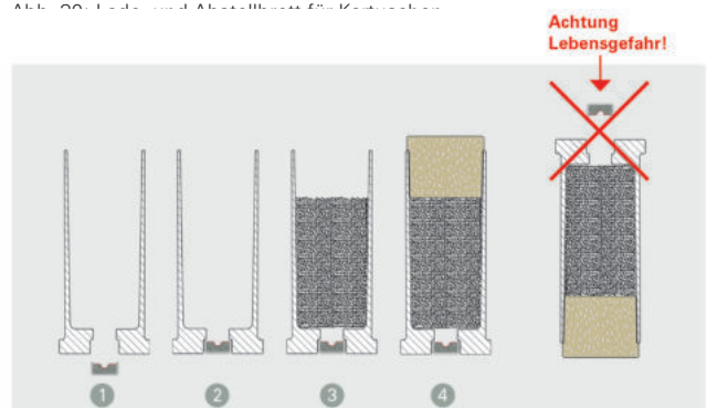
Abb. 31: Reihenfolge beim Laden einer Kartusche
